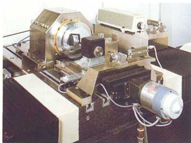
Bild 1. Ultrapräzisionsdrehmaschine UPM1. (Bild: IPT)
